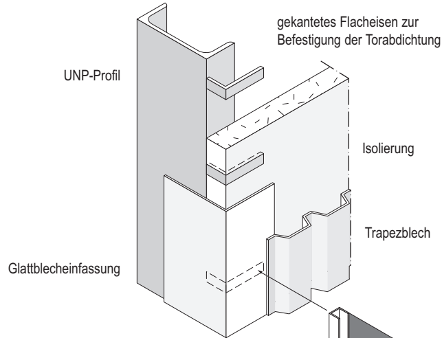
Schnitt C
