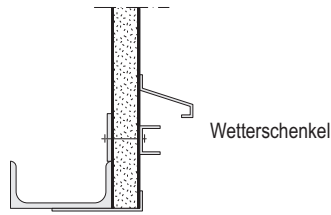
Schnitt A
