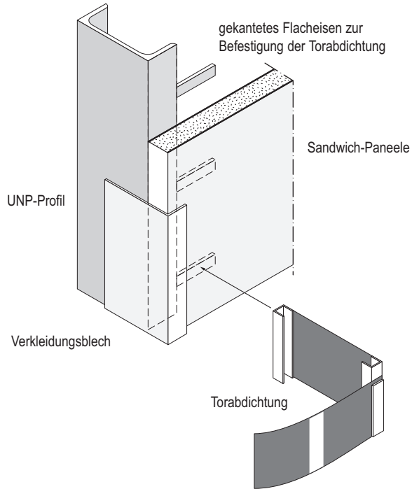
Ansicht D
