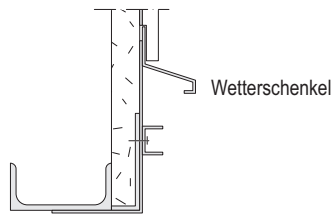
Schnitt A
