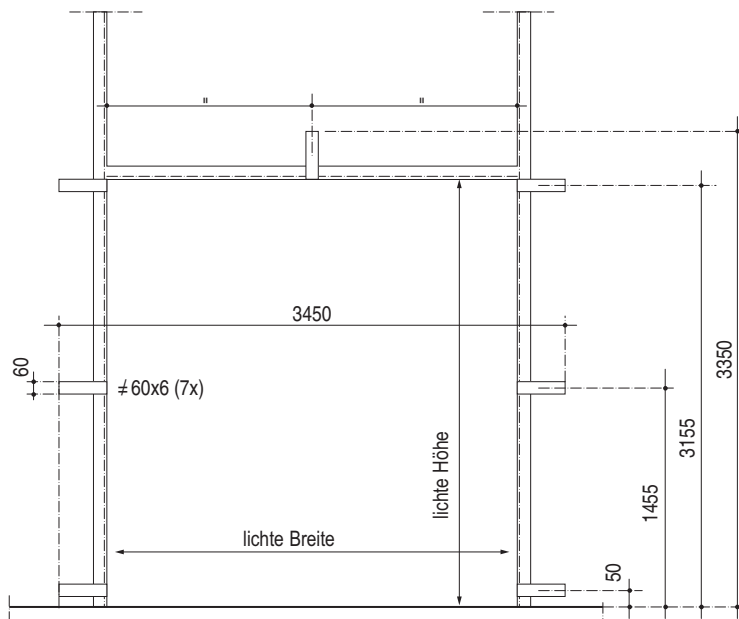
Bauseitige Voraussetzungen zur Befestigung der Torabdichtung (von Außen gesehen)
